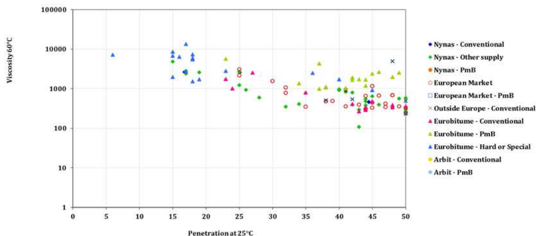
Figuur 5: Penetratie i.f.v. viscositeit voor verschillende penetratie bitumen.
